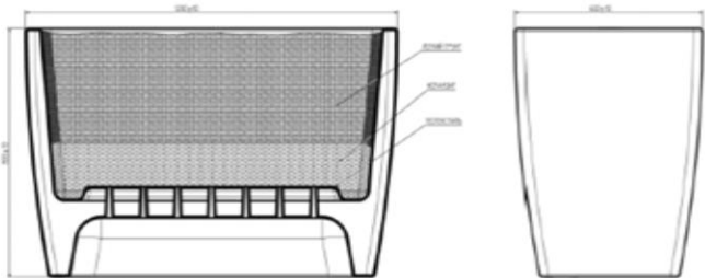
Чертеж МАФ
